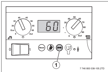
Fig. 16 Panoul de comandă al controlerului de bază
