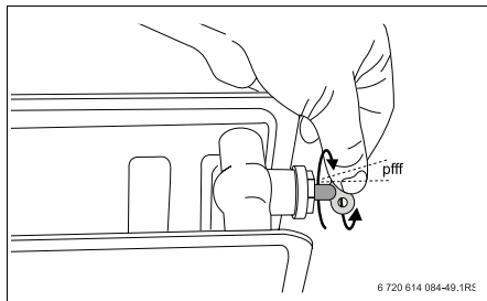
Fig. 14 Aerisirea radiatoarelor
