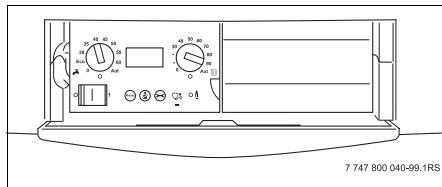
Fig. 3 Panoul de comandă de la nivelul controlerului de bază
