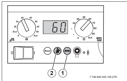
Fig. 8 Panoul de comandă al controlerului de bază
