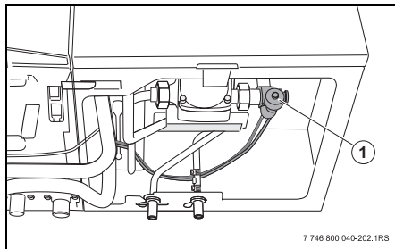
Fig. 15 Golirea rezervorului cu încărcare etapizată
