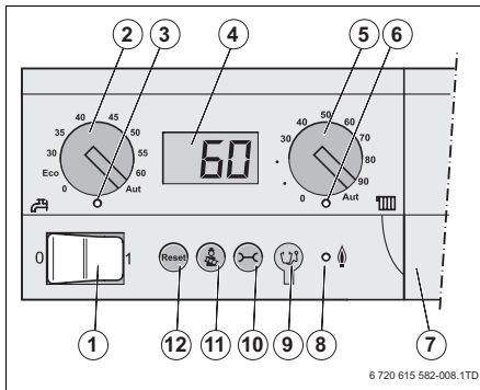
Fig. 5 Panou de comandă - Elemente de comandă
