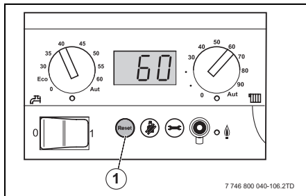
Fig. 17 Controler de bază BC10
