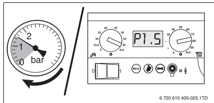
Fig. 10 Indicator de presiune analog/digital
